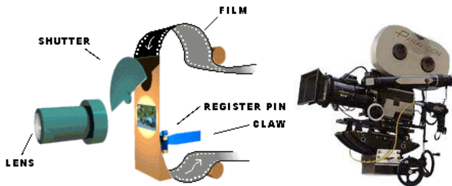
Mécanisme de l'obturateur
